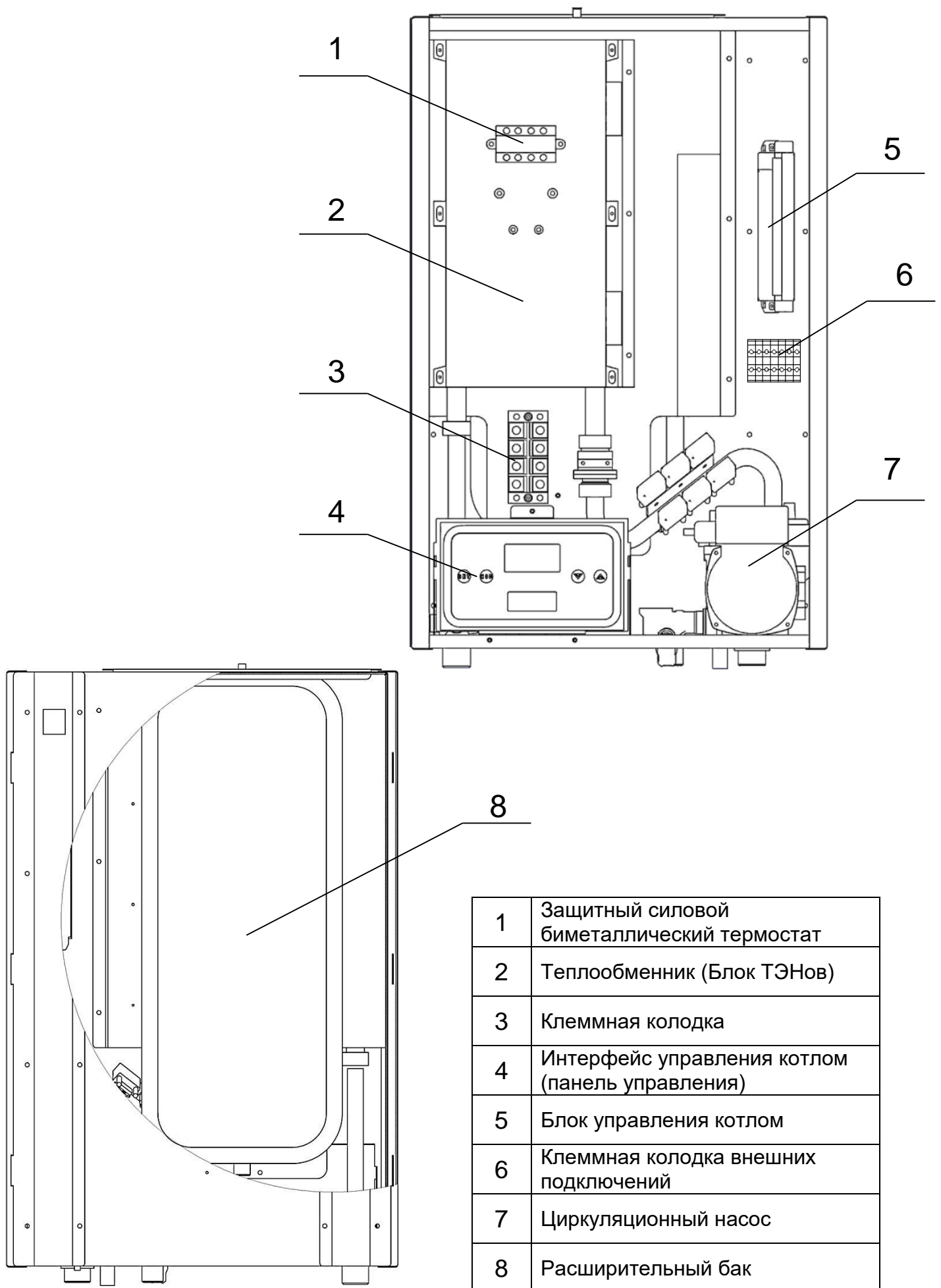
Рис. 2 Внутренне устройство
