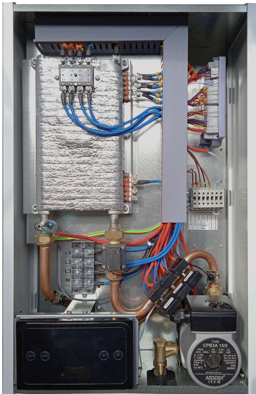
Рис. 1 Общий вид
