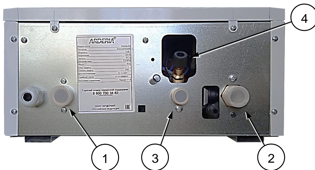
Рис. 17 Патрубки присоединения электродвигателя к трубам 1. выход ОВ из электродвигателя «подача»; 2. вход ОВ в электродвигатель «обратка»; 3. вход ХВС в электродвигатель; 4. кран подпитки
