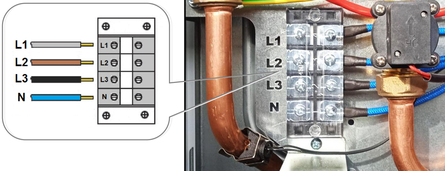
Рис. 14 Трёхфазное подключение
