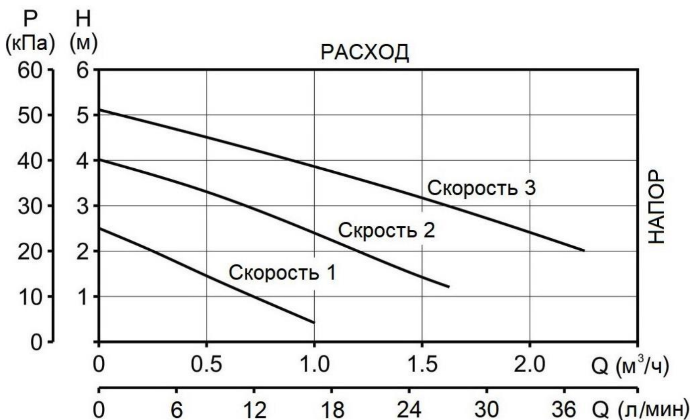
Рис. 19 Напорно-расходные кривые циркуляционного насоса электродкотла.
