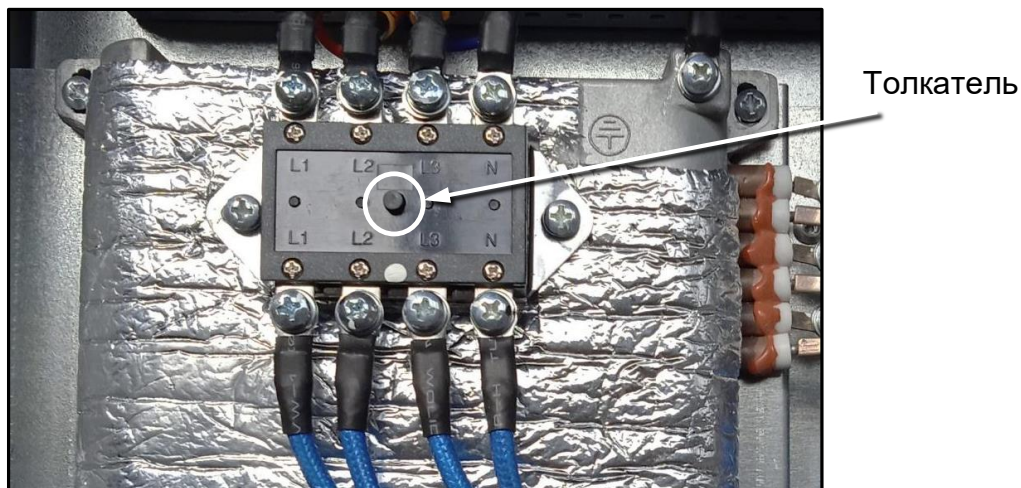
Рис. 8 Силовой биметаллический термостат (датчик перегрева)
